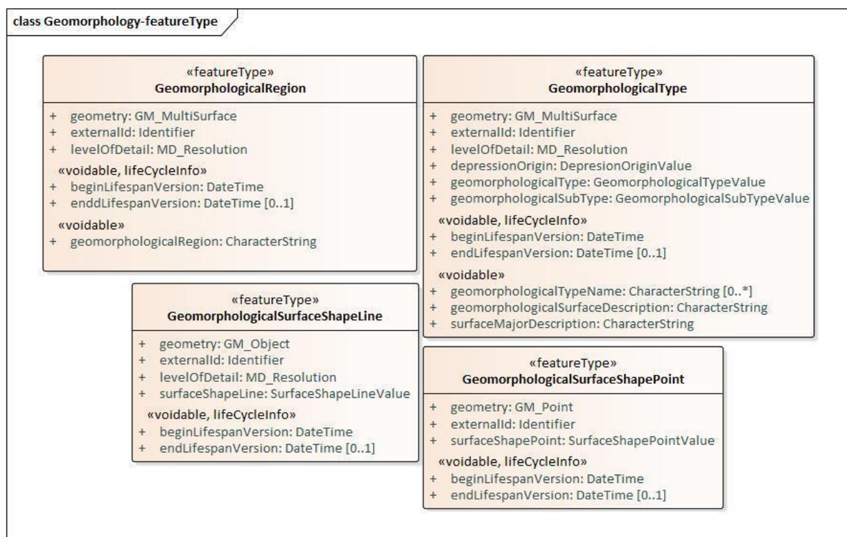
С.9-р зураг - UML диаграмм: “Геоморфологи (Geomorphology)” багцын биет төрлүүд
