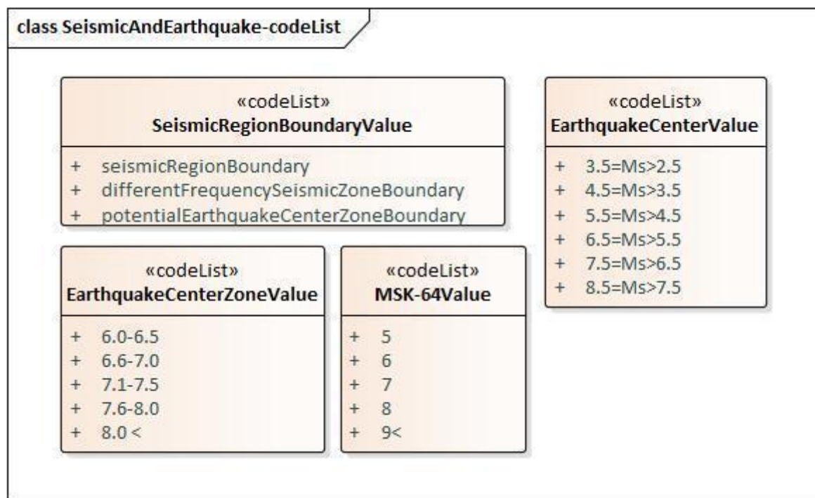
С.13-р зураг - UML диаграмм: “Газар чичирхийлэл, газар хөдлөл (Seismic and earthquake)” багцын кодын жагсаалт
