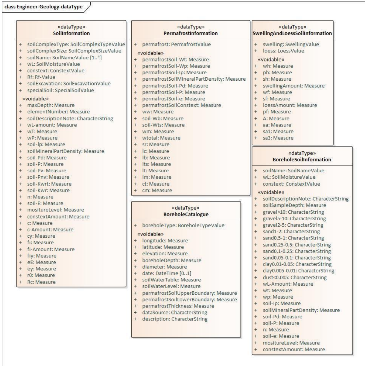
С.3-р зураг - UML диаграмм: “Инженер-геологи (Engineering geology)” багцын өгөгдөл төрлүүд
