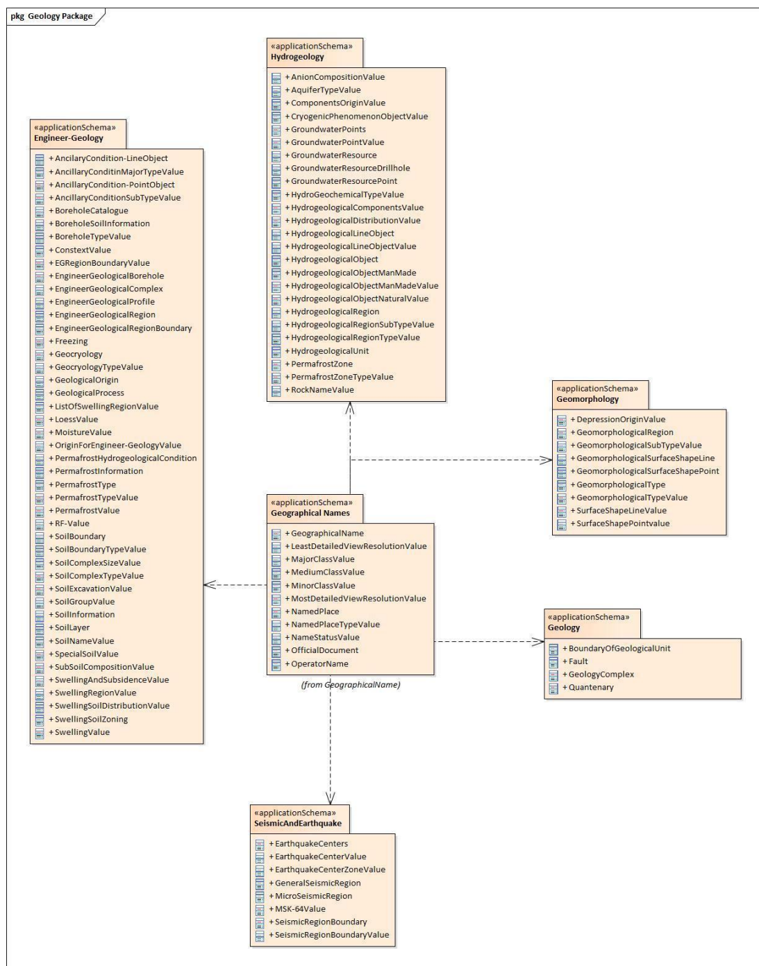
С.1- зураг - UML диаграмм: “Инженер-геологийн өгөгдлийн үзүүлэлт” хэрэглээний тойм схем
