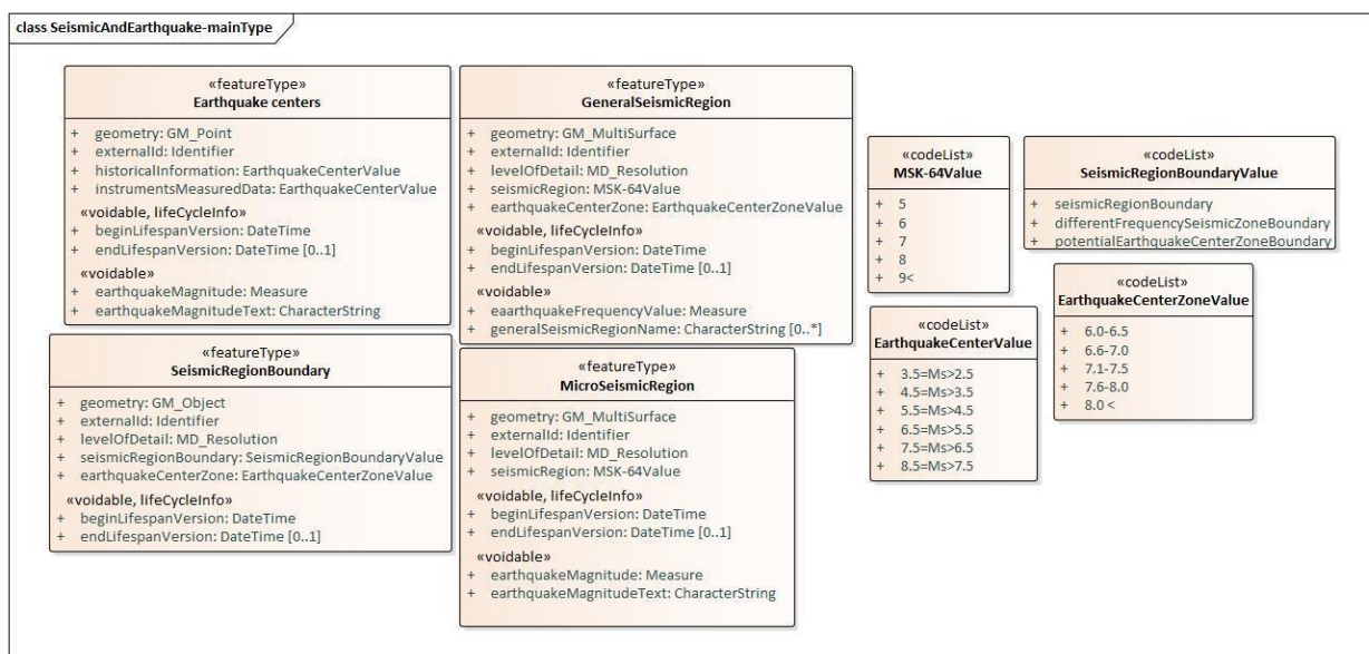
С.11-р зураг - UML диаграмм: “Газар чичирхийлэл, газар хөдлөл (Seismic and earthquake)” багцын хэрэглээний тойм схем
