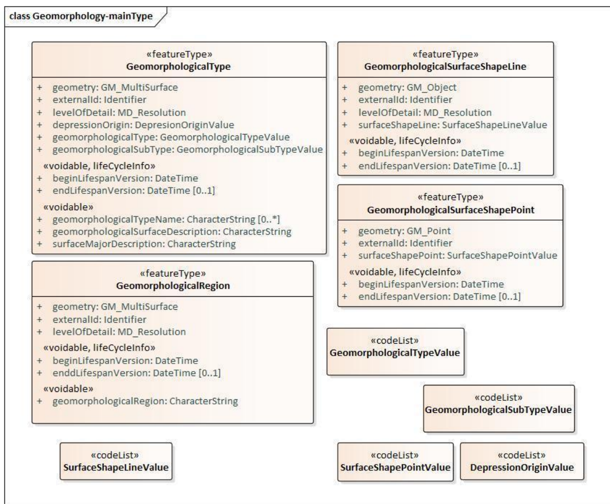
С.8-р зураг - UML диаграмм: “Геоморфологи (Geomorphology)” багцын хэрэглээний тойм схем
