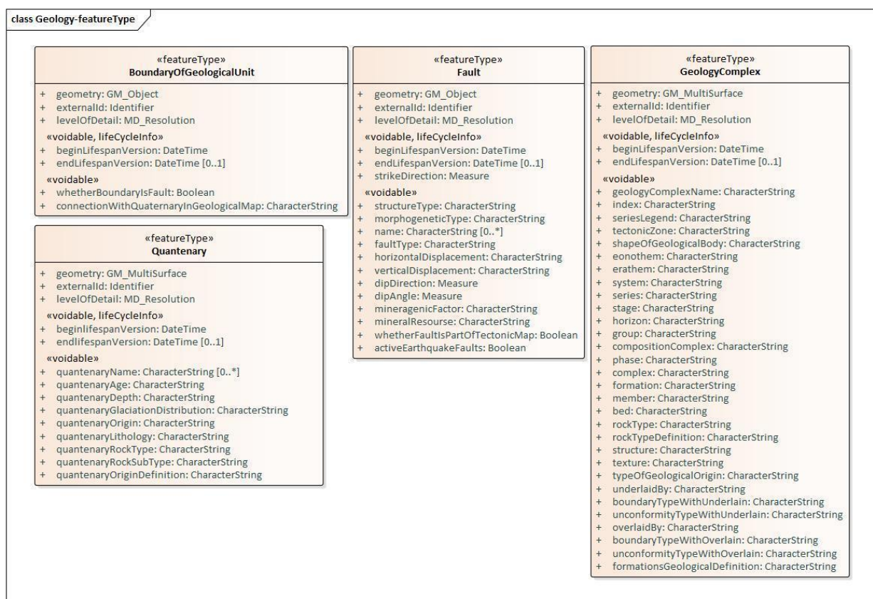
С.14-р зураг - UML диаграмм: “Геологи (Geology)” багцын биет төрлүүд
