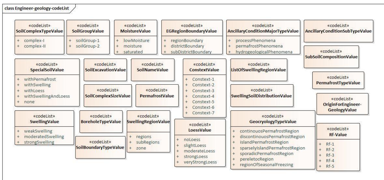
С.4-р зураг - UML диаграмм: “Инженер-геологи (Engineering geology)” багцын кодын жагсаалт
