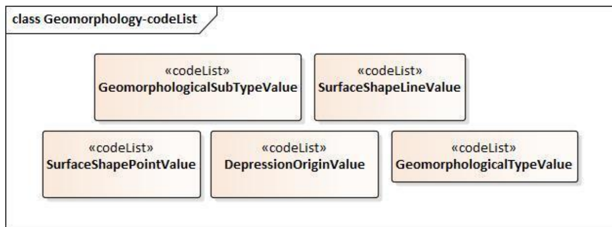
С.10-р зураг - UML диаграмм: “Геоморфологи (Geomorphology)” багцын кодын жагсаалт
