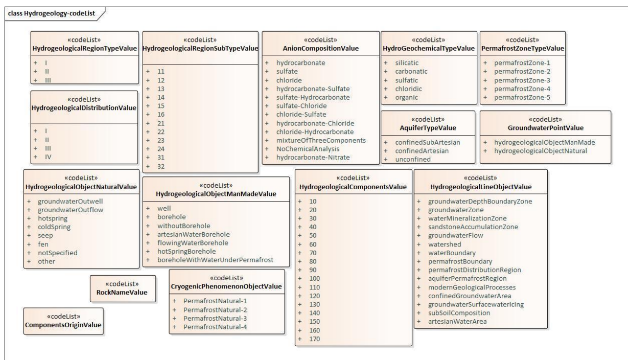
С.7-р зураг - UML диаграмм: “Гидрогеологи (Hydrogeology)” багцын кодын жагсаалт
