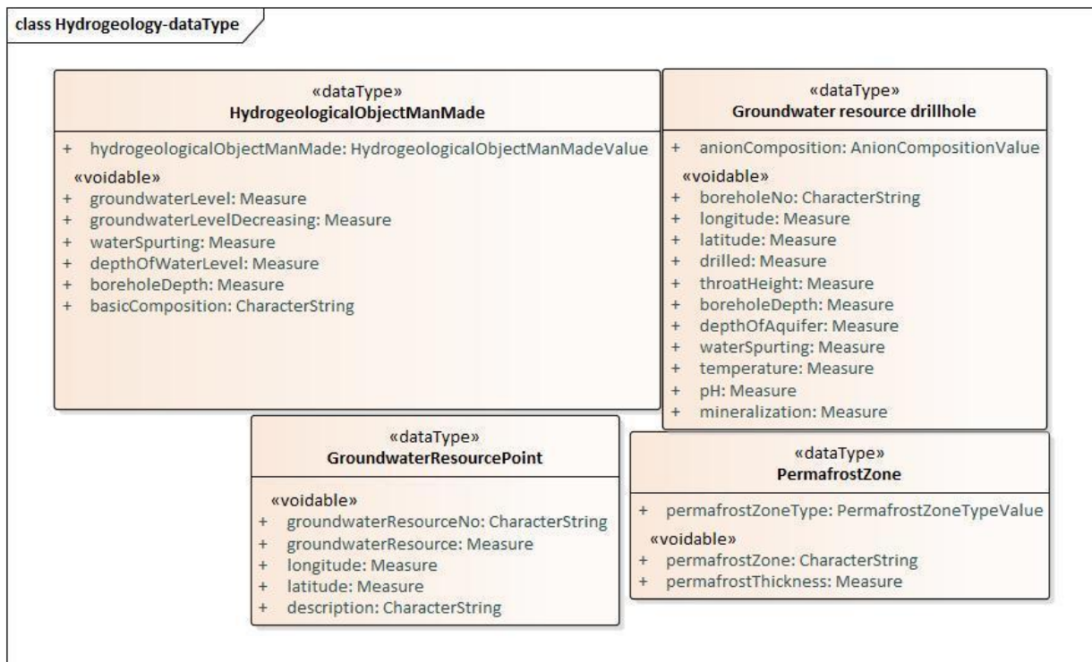
С.6-р зураг - UML диаграмм: “Гидрогеологи (Hydrogeology)” багцын өгөгдөл төрлүүд
