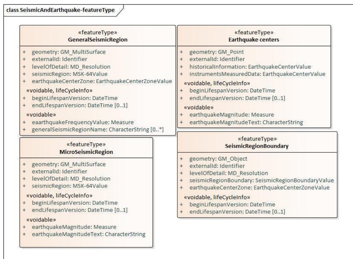
С.12-р зураг - UML диаграмм: “Газар чичирхийлэл, газар хөдлөл (Seismic and earthquake)” багцын биет төрлүүд
